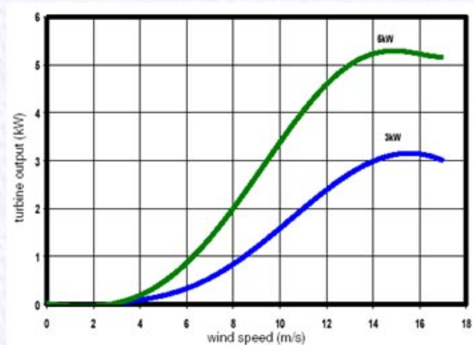
功率曲線圖
