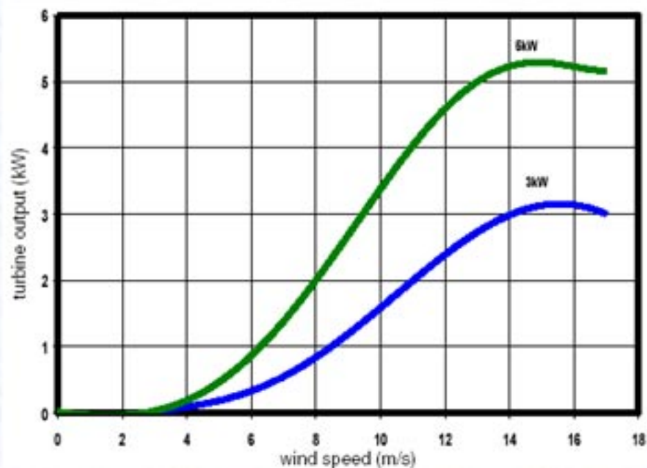
功率曲線圖
