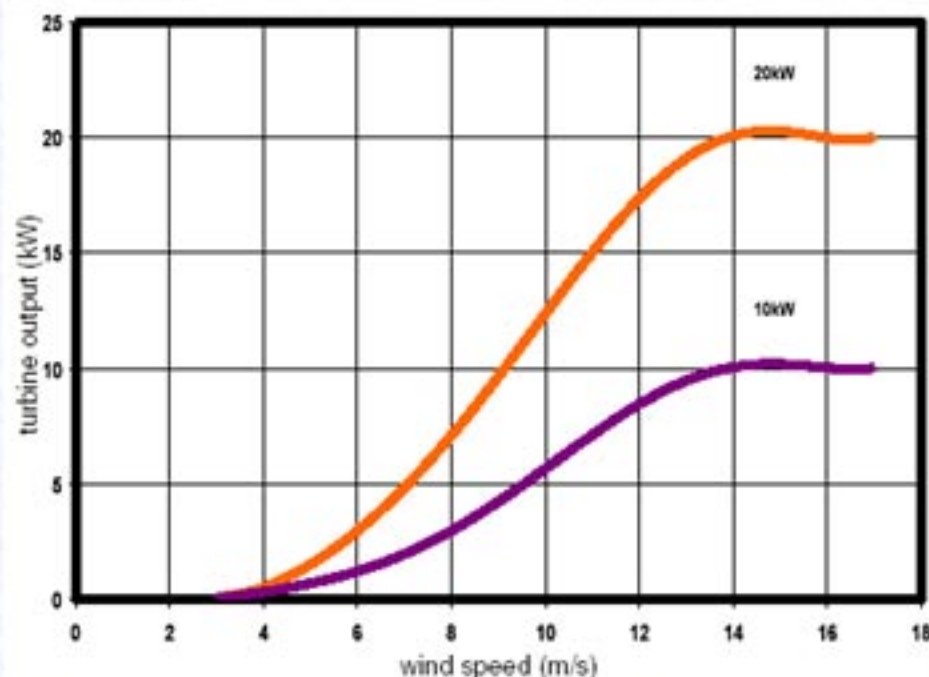
功率曲線圖
