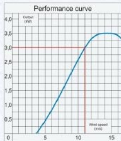
功率曲線圖
